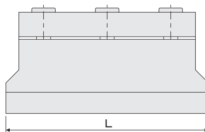
切斷板座 Tool Block
