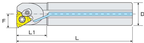
右車刀桿圖示 Right-Hand Shown
